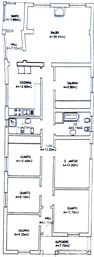
PLANTA DA MORADIA
